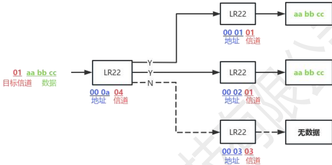
图 3：广播传输
