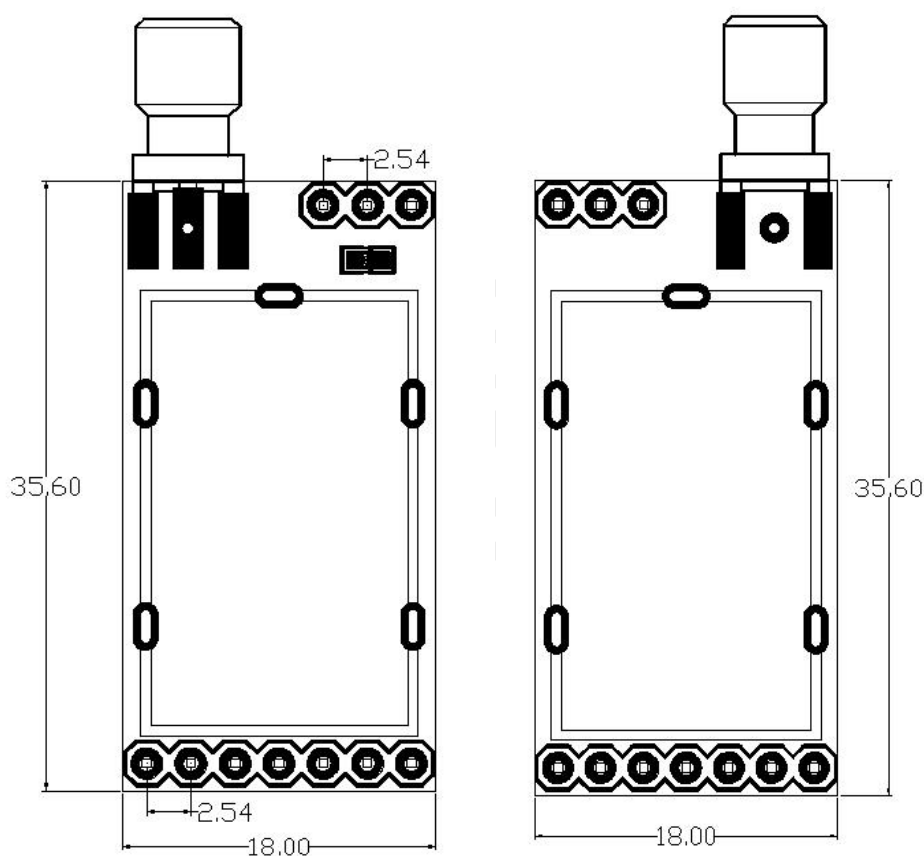
图 8：模块俯视及底视尺寸图
